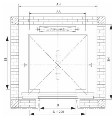
MẶT CẮT NGANG GIẾNG THANG
