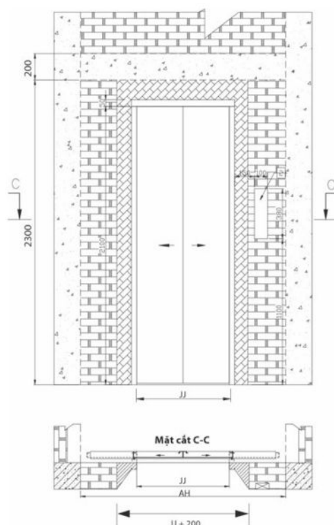
ĐỐI TRỌNG PHÍA SAU, CỬA MỞ TIM
